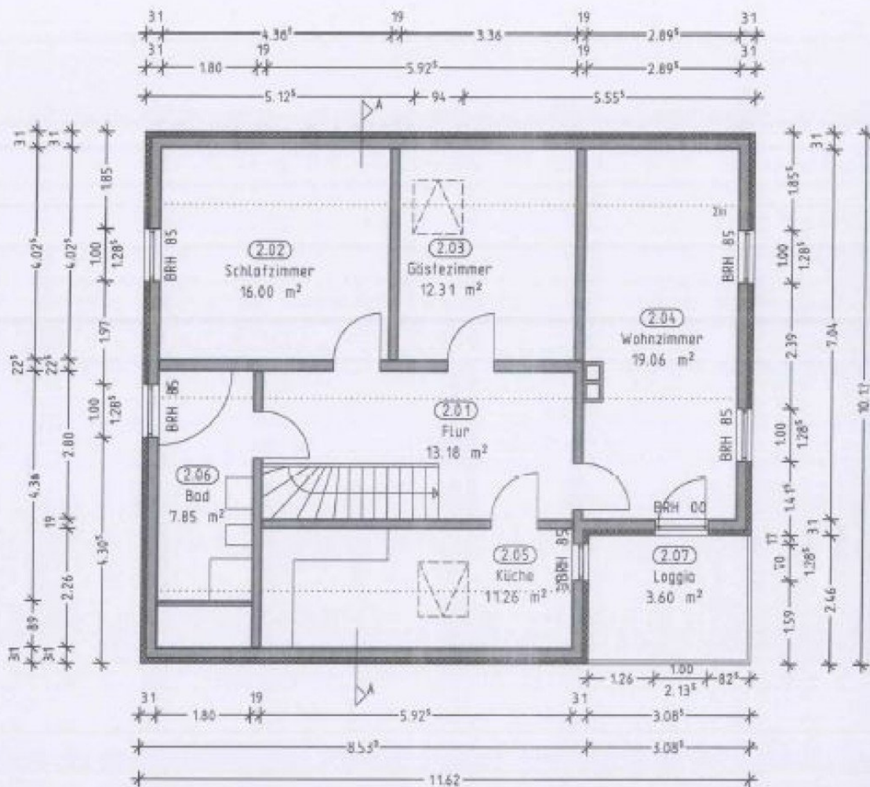
Grundriss DG
