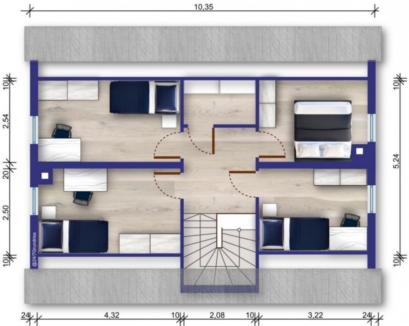
Grundriss DG
